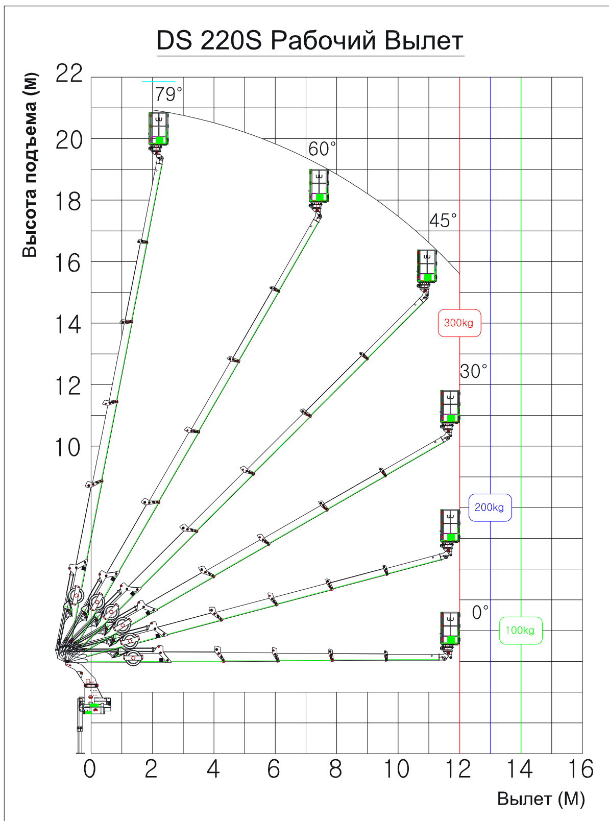
Зона обслуживания при работе с рабочей платформой в вертикальной плоскости
