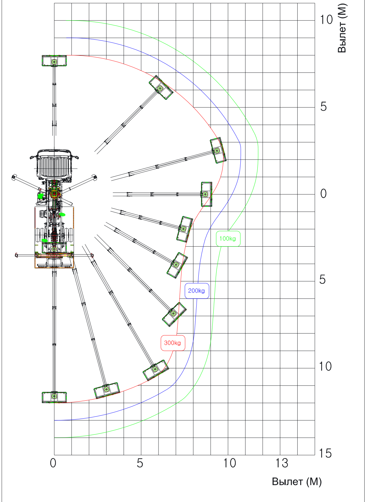
Зона обслуживания при работе с рабочей платформой в горизонтальной плоскости
